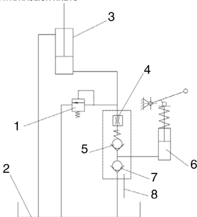
Fig.5: Hydrauliskt diagram
